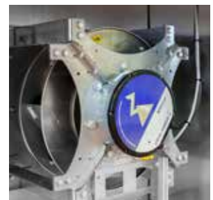
Roue libre avec moteur à commutation électronique
